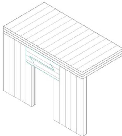
Dintel
